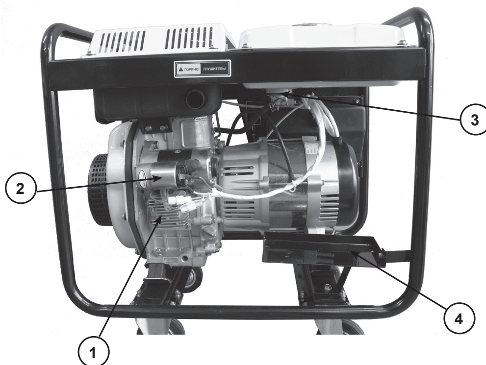
1. Регулятор зарядки АКБ 2. Стартер электрический 3. Кран топливный 4. Отсек АКБ
