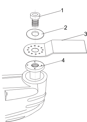
Установка ножа
