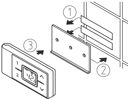
Рис. А. Установка с помощью клейкой ленты
