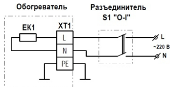
Рис. 2 Схема подключения обогревателя IRC-08, IRC-10; IRC-15
