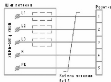
Рис. 3 Схема подключения розетки к стационарной сети
