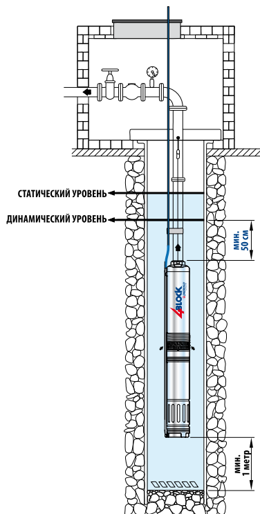
Типовая схема установки
