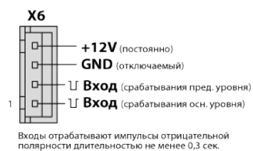
Подключение дополнительного датчика
