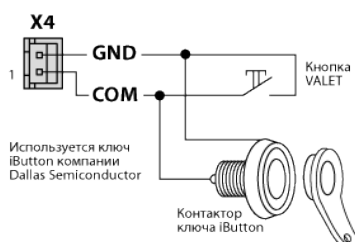
Подключение контактора ключа iButton
