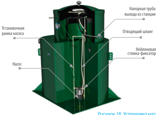
Рисунок 18. Установка насоса удаления воды камеры чистой воды.
