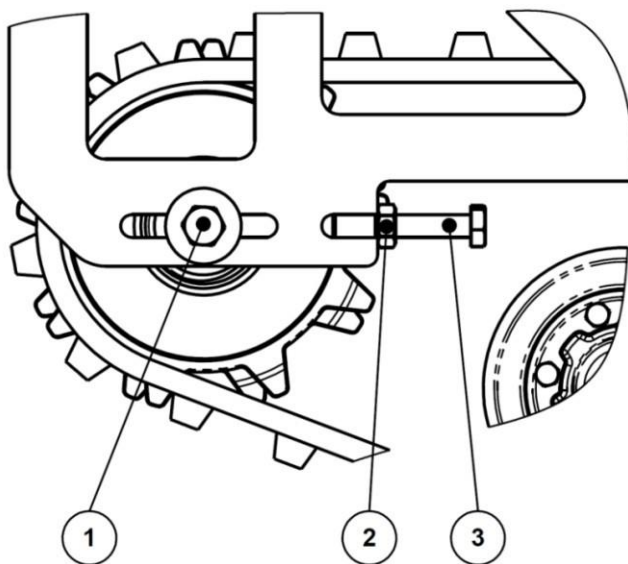
Рис.5 Натяжение гусеницы
