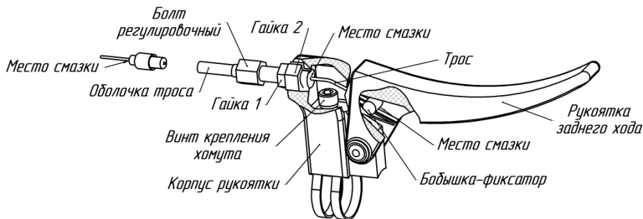
Рис.7 Заделка троса в ручьятке газа
