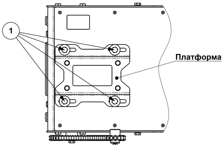
Рис.4 Способ натяжения цепи
