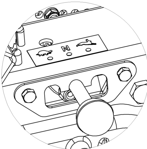
Рис.6 Рычаг удвоителя.
