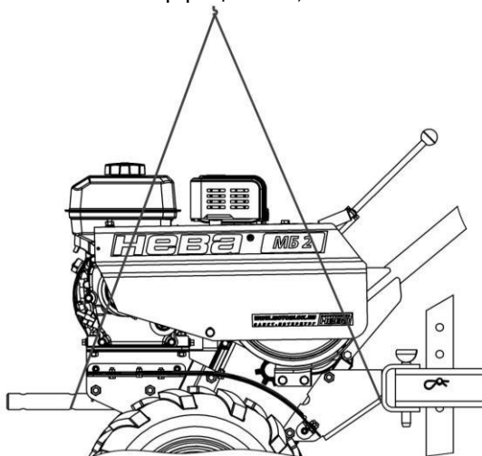
Рис.4. Схема зачаливания мотоблока при погрузке.
