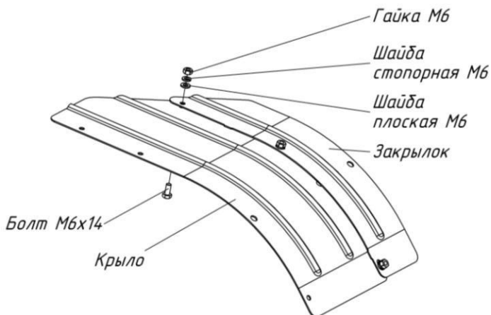
Рис.3. Схема крепления закрывков (дополнительных крыльев)
