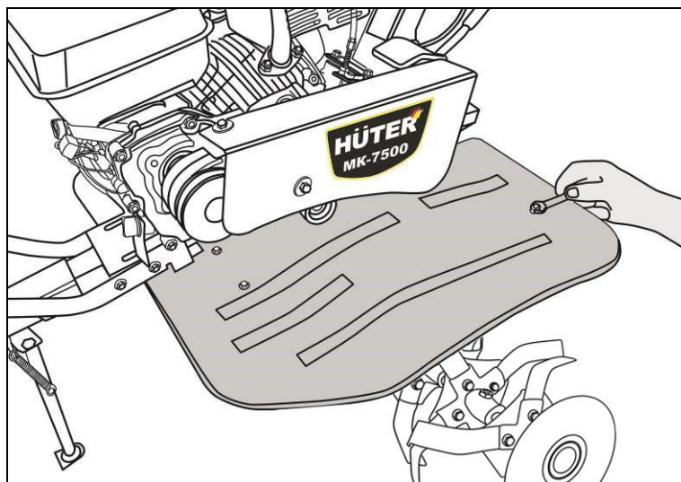
Рис.16. Фиксация крыльев
