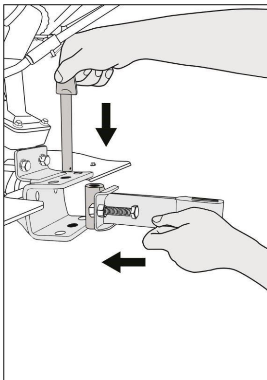
Рис.17. Установка сцепки
