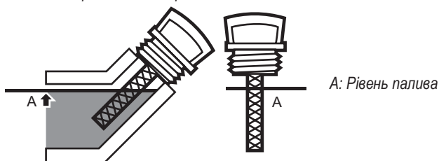
Рис. 1. Вимірювальний стрижень.
