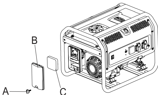
Рис. 8. Повітряний фільтр
