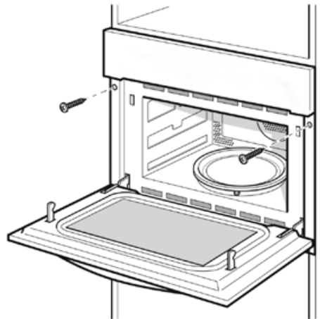
Крепление духового шкафа к мебели.
