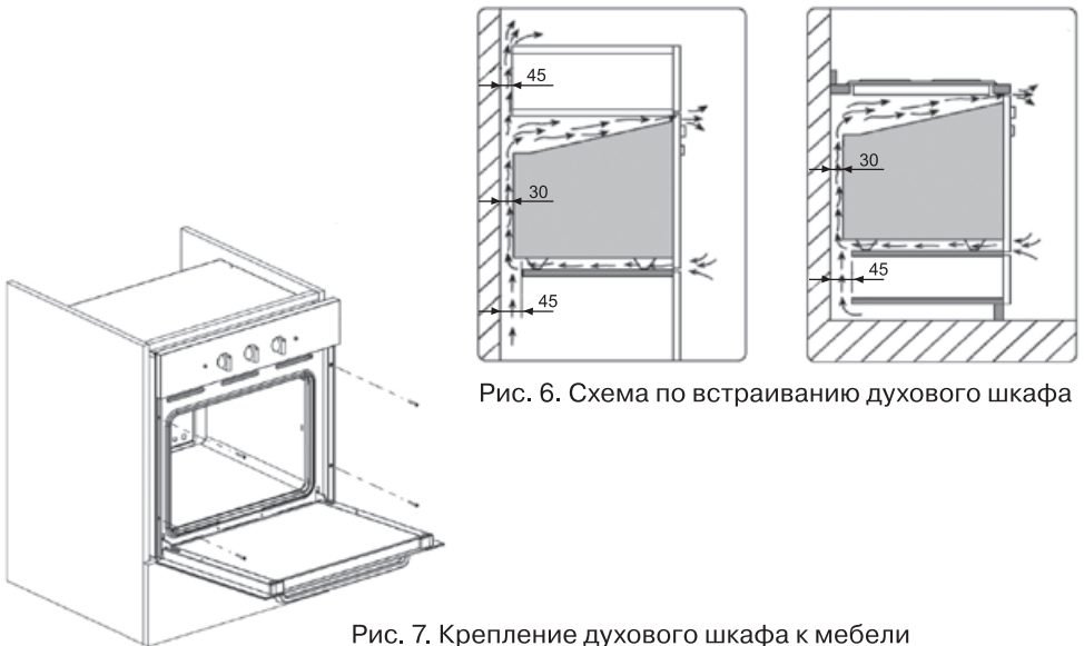
Рис. 7. Крепление духового шкафа к мебели
