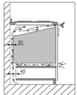
Рис. 6. Схема по встраиванию духового шкафа
