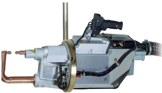
Клещи 3323 с блоком ТЕ450
