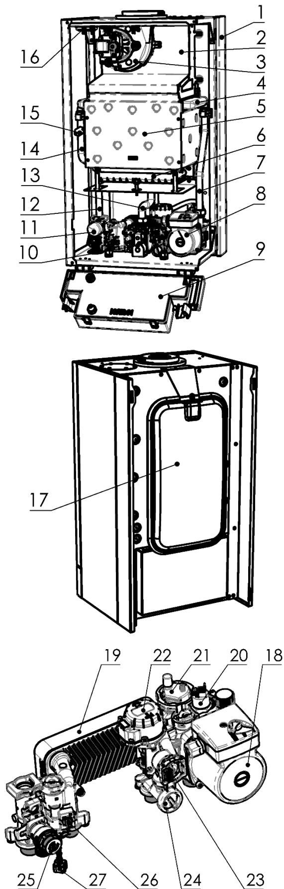
Рис. 10. Общая схема и основные элементы котла
