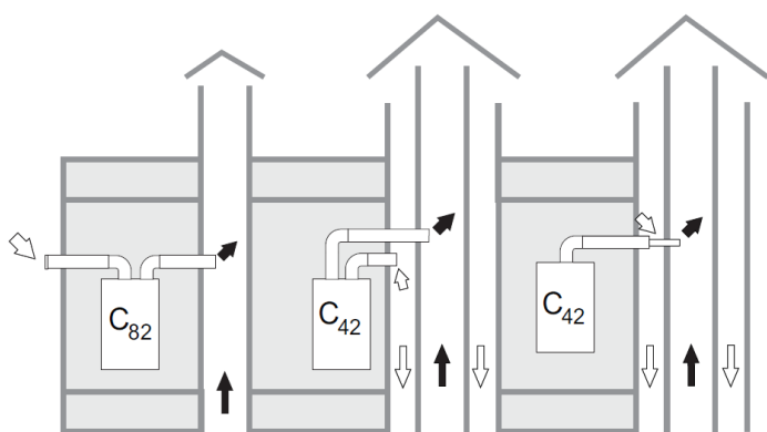
Рис. 6. Примеры систем дымоудаления собранных с помощью раздельных труб. Белой стрелкой обозначен приток воздуха, чёрной стрелкой поток продуктов сгорания.
