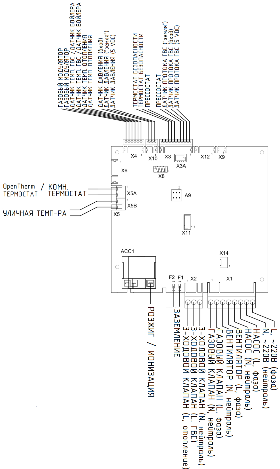
Рис. 14. Электрическая схема
