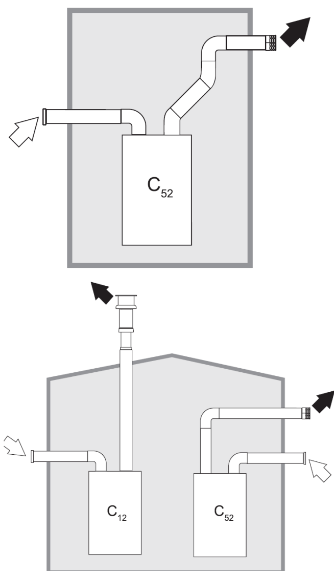
Рис. 4. Пример систем дымоудаления собранных с помощью отдельных труб. Белой стрелкой обозначен приток воздуха, чёрной стрелкой отвод продуктов сгорания
