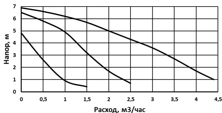
Рис. 13. Напорная характеристика насоса.
