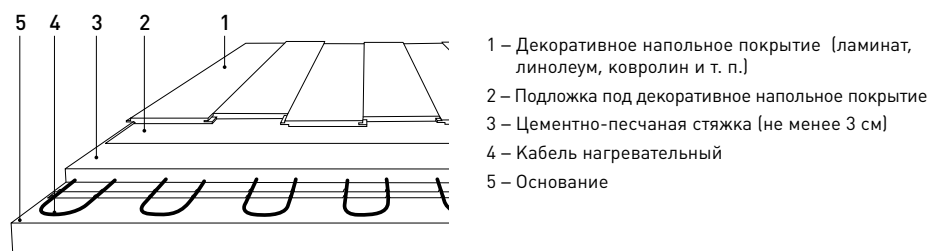
Схема укладки под ламинат, линолеум или ковролин
