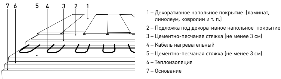
Схема укладки под ламинат, линолеум или ковролин в холодных помещениях
