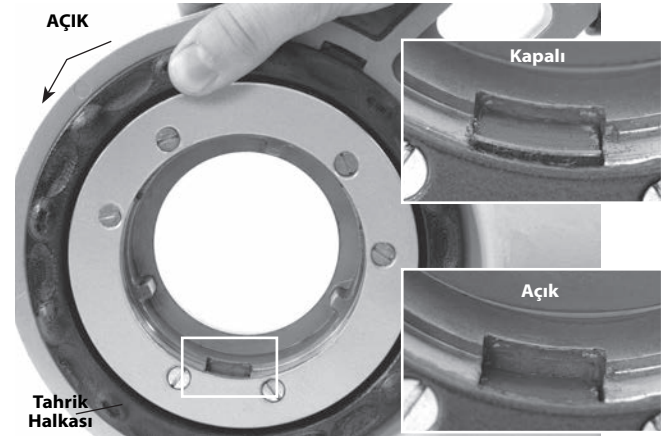
Şekil 7 - Tespit Mekanizması, Tahrik Halkası Açık/Kapalı Konumda
