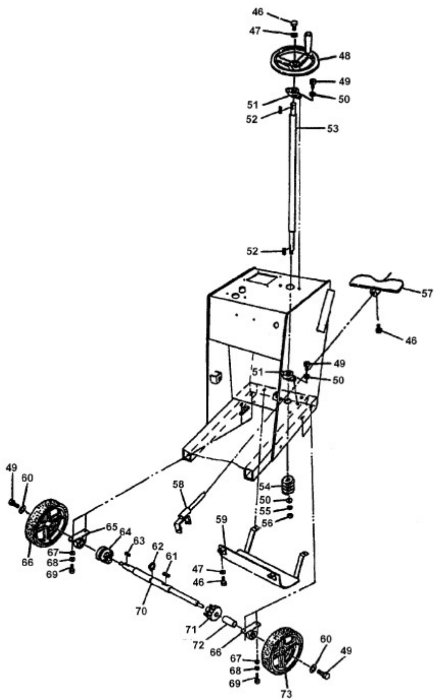
КОРОБКА ПЕРЕДАЧ
