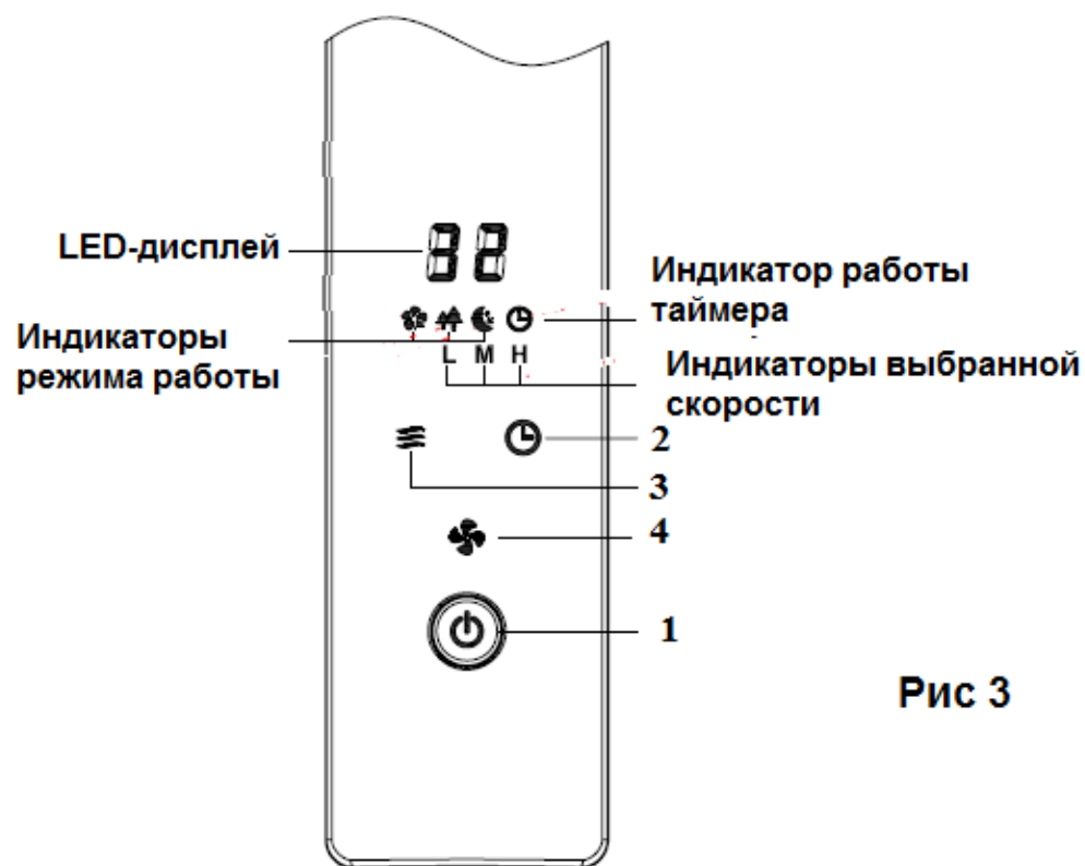
Панель управления
