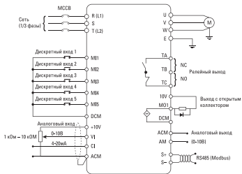
Рис. 6. Схема подключения преобразователей частоты VECTO100 от 0,4 до 2,2 кВт
