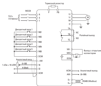
Рис.7. Схема подключения преобразователей частоты VECTO100 от 4 до 7,5 кВт
