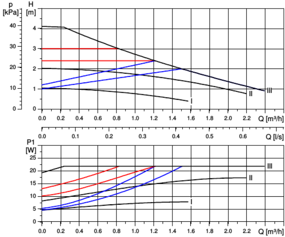
Рис. 16 Кривые рабочей характеристики, ALPHA2 L XX-40
