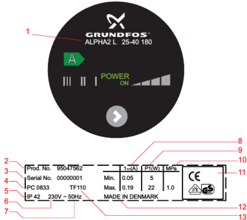
Рис. 19 Фирменная табличка, GRUNDFOS ALPHA2 L
