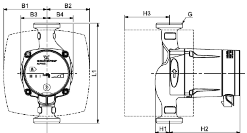
Рис. 14 Габаритные чертежи, ALPHA2 L XX-40, XX-50, XX-60
