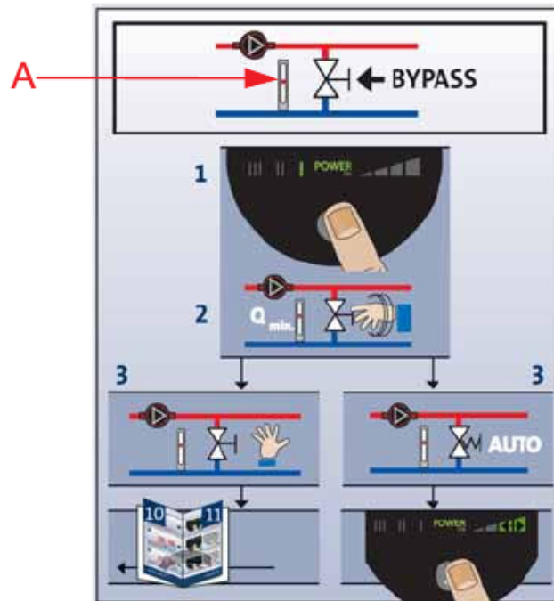
Рис. 10 Системы с перепускным клапаном
