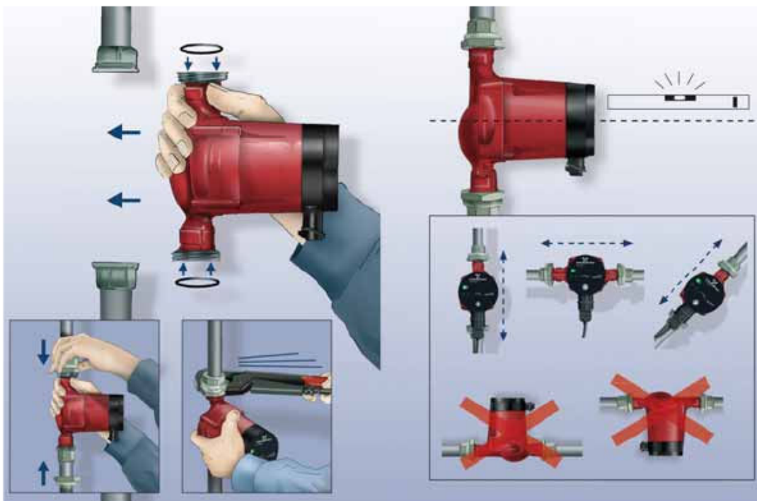
Рис. 3 Монтаж GRUNDFOS ALPHA2 L
