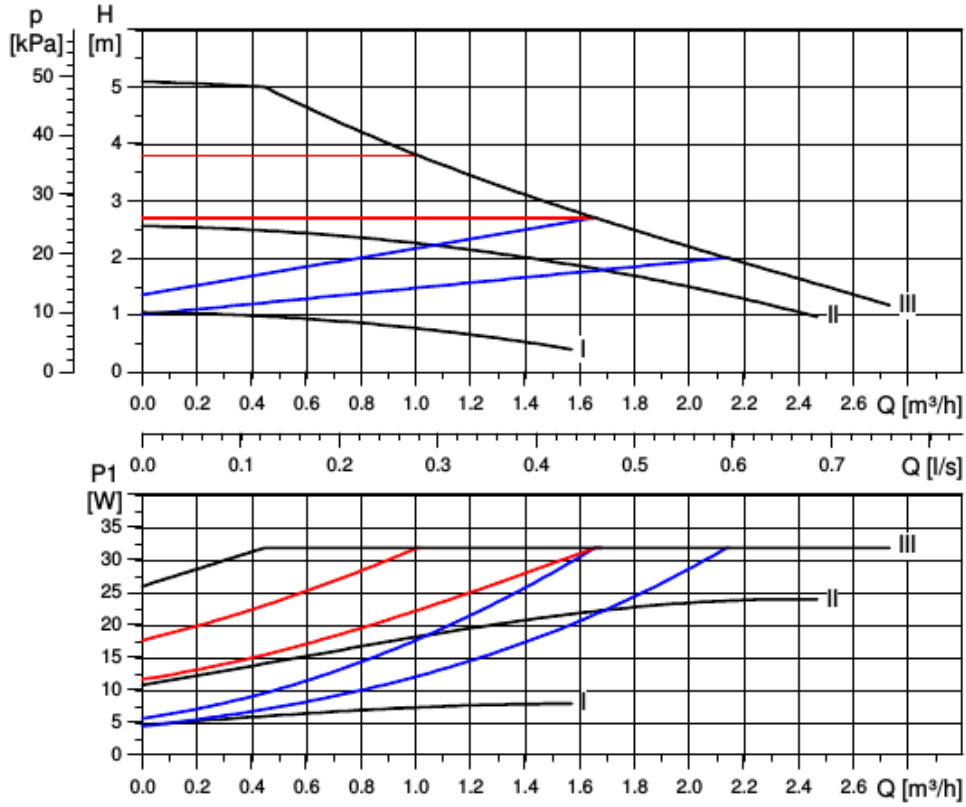
Рис. 17 Кривые рабочей характеристики, ALPHA2 L XX-50
