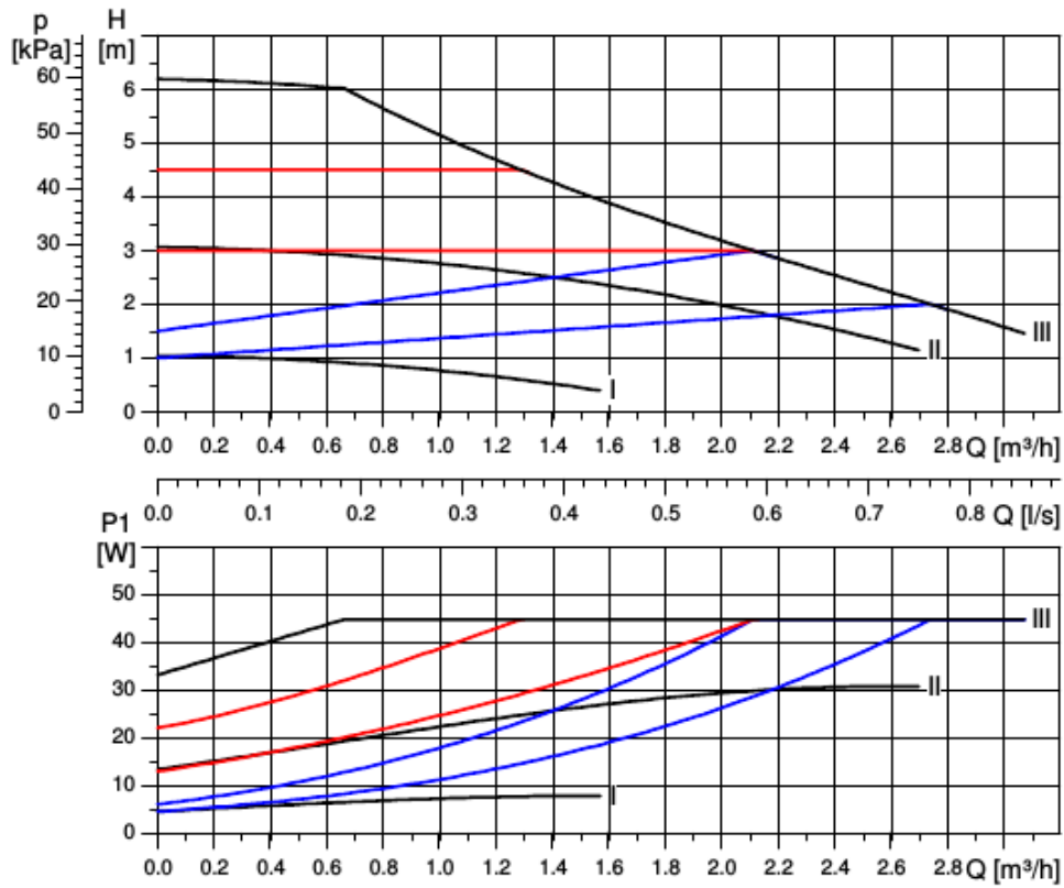
Рис. 18 Кривые рабочей характеристики, ALPHA2 L XX-60
