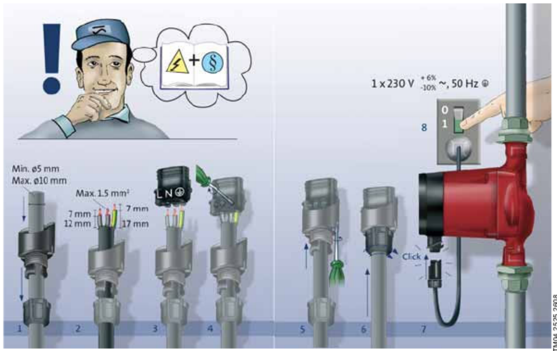
Рис. 6 Подключение электрооборудования
