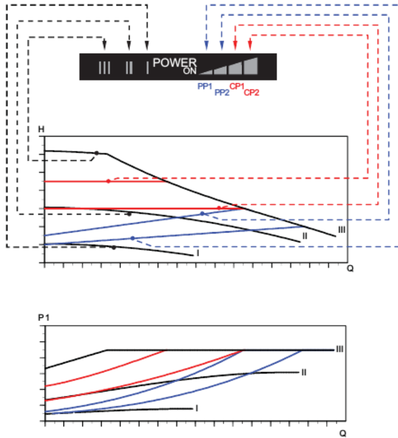
Рис. 15 Соотношение между настройками насоса и рабочими характеристиками
