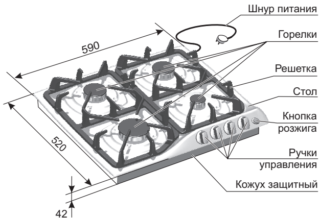
Рис. 1 МОДЕЛЬ СН1210
