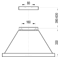
Схема установки для модели AVEX YS 6040 X
