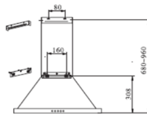
Схема установки для моделей AVEX RYS 6040 Y / B
