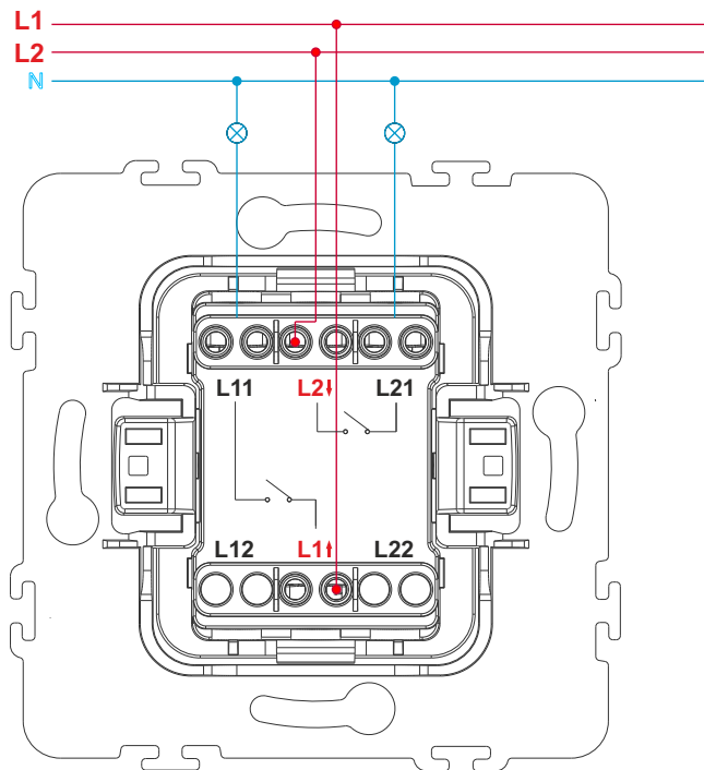
Вариант подключения двух фаз
