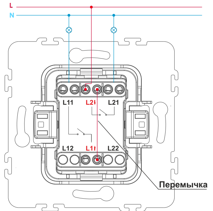
Вариант подключения одной фазы
