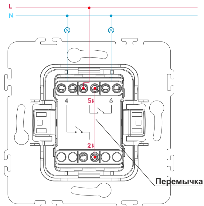
Вариант подключения одной фазы
