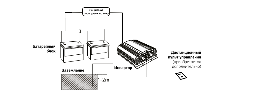
Рисунок 6.2: Подключение инверторов KV-M1000/KV-M1500/KV-M2000/KV-M2500/ KV-P1000/KV-P1500/KV-P2000/KV-P3000
