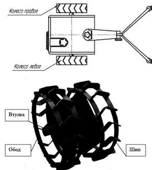
Рис.1. Схема установки грунтозацепов на культиватор
