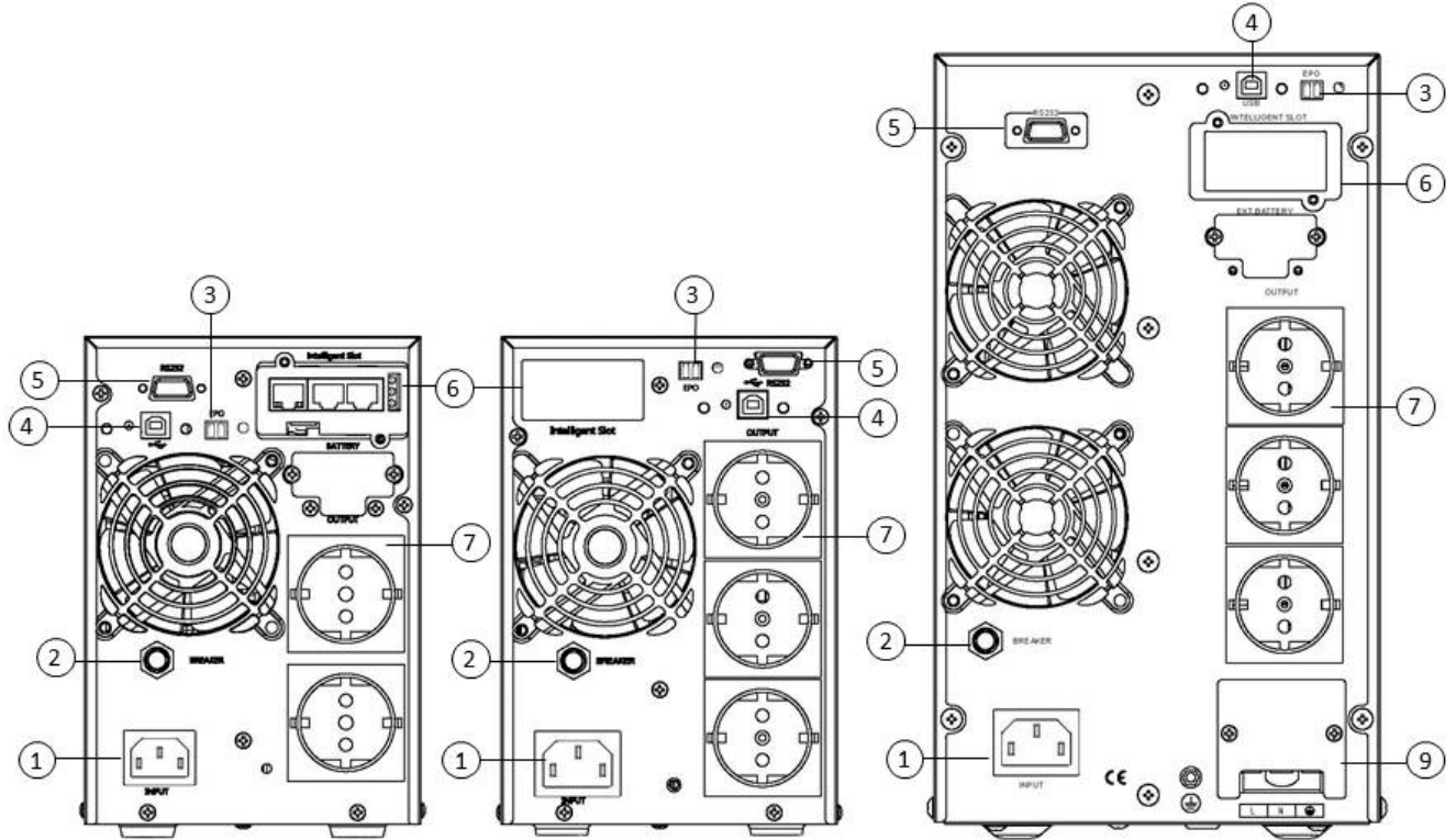
Рис.2 Задняя панель ИБП серии ONLINE 1000/2000/3000.
