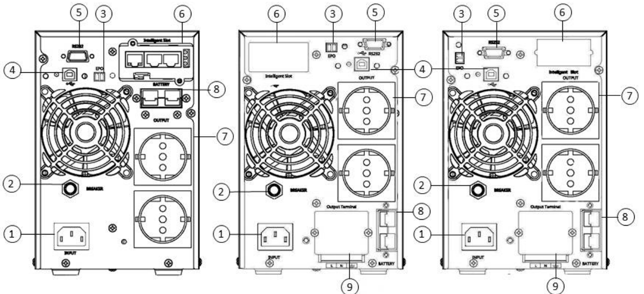
Рис.3 Задняя панель ИБП серии ONLINE PLUS 1000/2000/3000.
