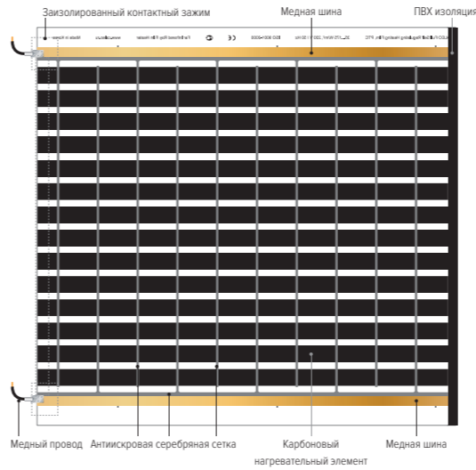
Рис. Общий вид термопленки CALEO, расположение основных ее элементов, контактных зажимов и мест подключения и изоляции
