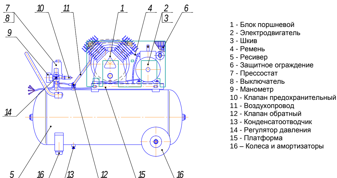
Рисунок 7 - Общий вид компрессоров СБ4/С-100.LB30, СБ4/С-100.LB30А
