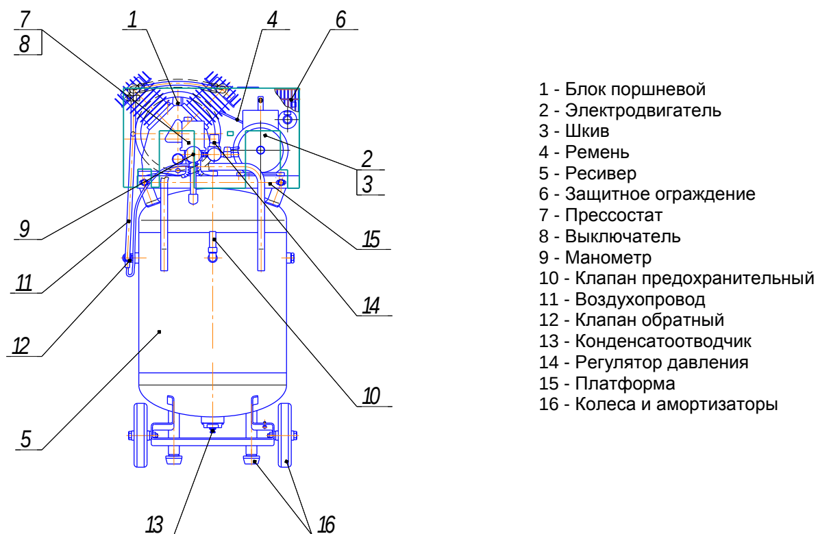
Рисунок 8 - Общий вид компрессоров СБ4/С-100.LB30В, СБ4/С-100.LB30АВ
