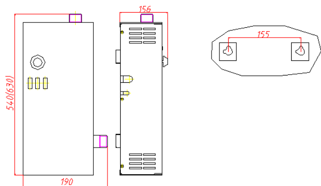
Рис.1 Электроводонагреватель.
