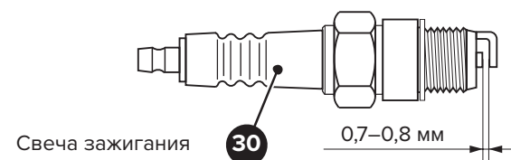
Рисунок 12 — Необходимый зазор в свече зажигания
