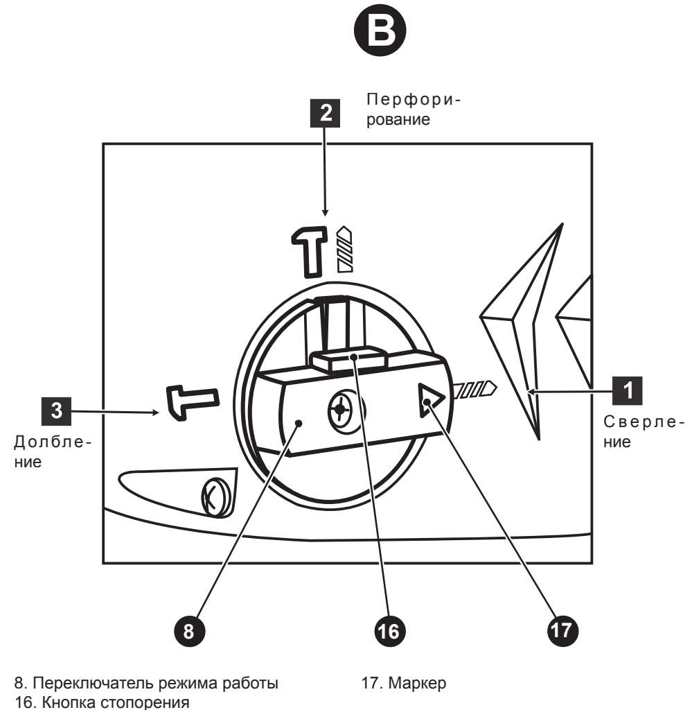
Рисунок В — положения переключателя перфоратора в зависимости от выбранного режима работы.
