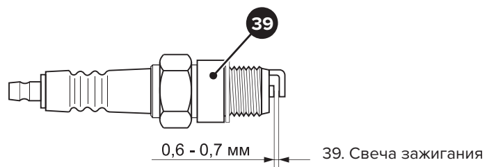
Рисунок 18 — Необходимый зазор в свече зажигания
