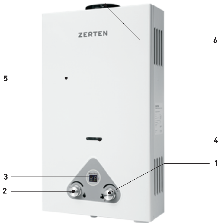
Рис. 1. Аппарат водонагревательный проточный газовый бытовой «ZERTEN» 1 - ручка водяного регулятора; 2 - ручка газового регулятора; 3 - цифровой индикатор температуры горячей воды; 4 - окно смотровое; 5 - облицовка; 6 - патрубок дымоотвода.
