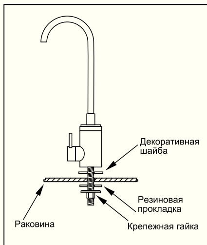
Рис. 5-3 Установка крана
