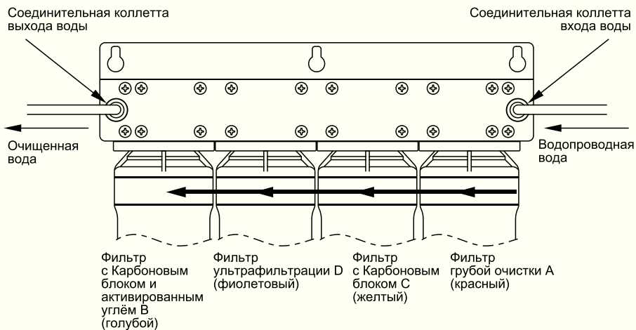
Рис. 1-2 Вид сзади
