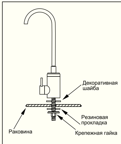
Рис. 5-3 Установка крана
