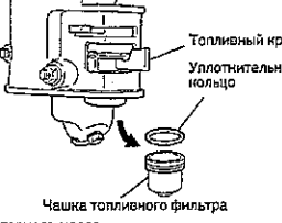
Чашка топливного фильтра
