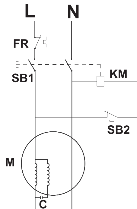
Рисунок А — принципиальная электрическая схема бетоносмесителя оснащенного электродвигателем 220 В.
