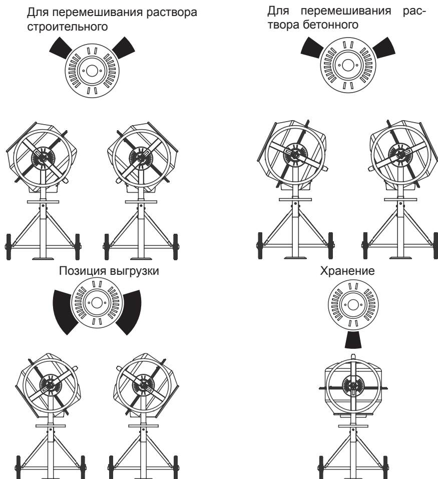
Рисунок Е — положения барабана бетоносмесителя при работе и хранении.
