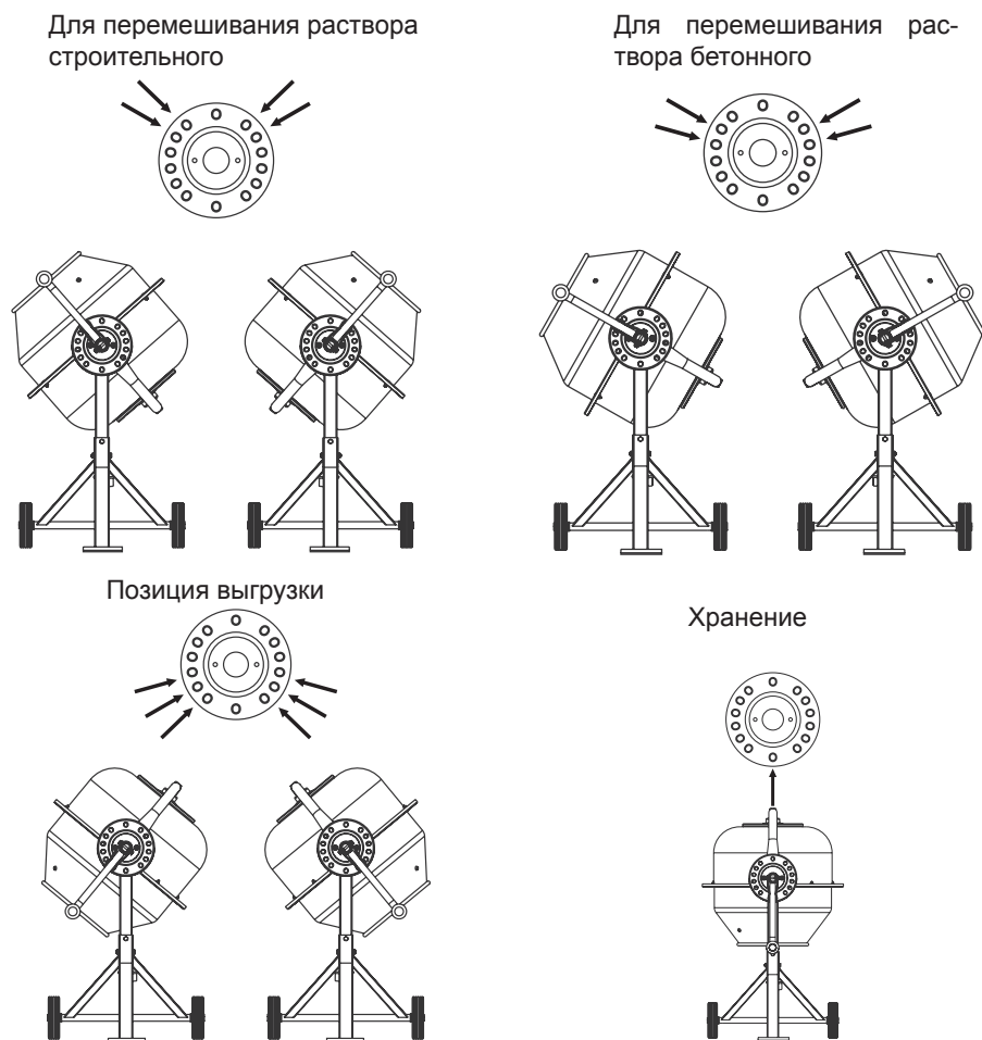
Рисунок Е — положения барабана бетоносмесителя при работе и хранении.
