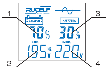
Рис. 1 Дисплей ИБП
