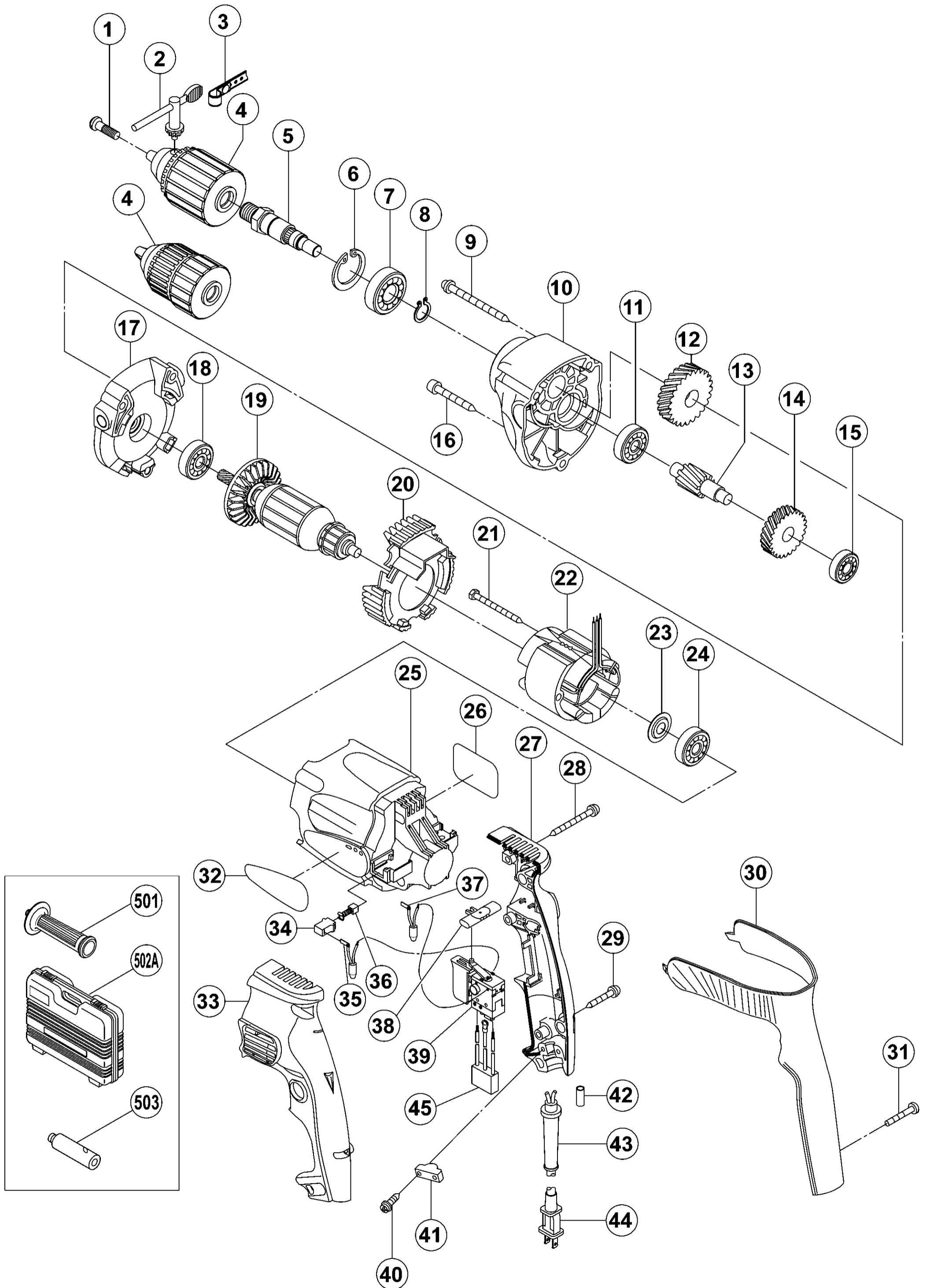
形 名 D13VF(1/2)
