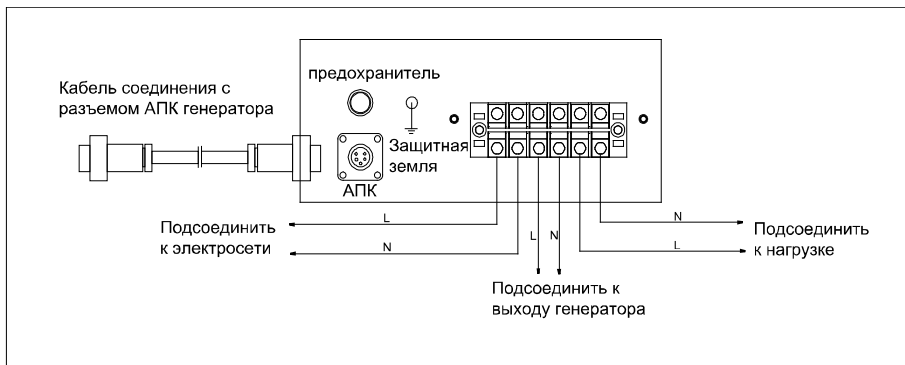
Рисунок 1. Схема подключения.
