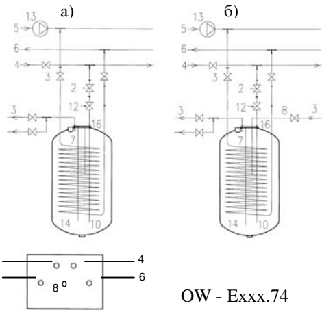
Рис. 5. Схема гидросистемы а) без циркуляции, б) с циркуляцией
