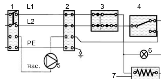
Рис. 3 Электросхема
