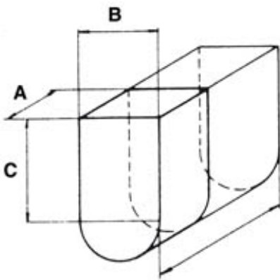
Параметры выборки цепной гарнитурой 28 x 40 x 100 мм, ширина цепи (A): 28 мм, ширина отверстия (B): 40 мм, глубина долбления (C): 100 мм
