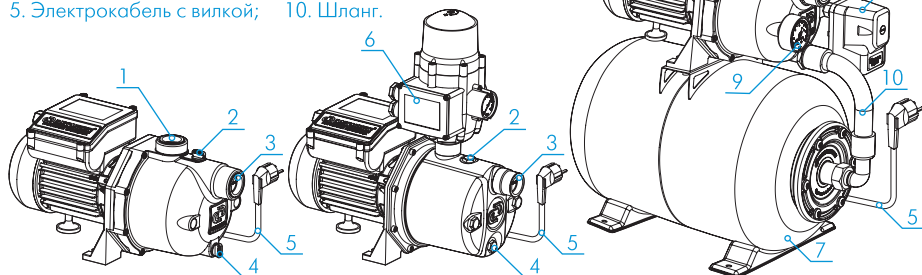
Поверхностный насос
