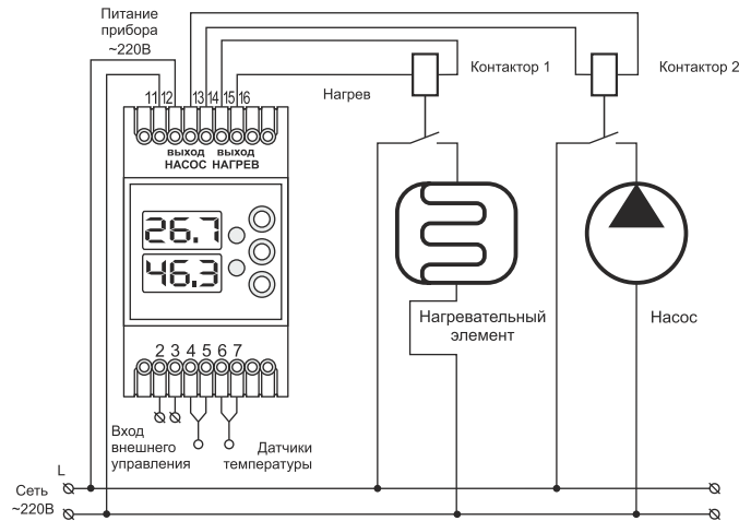
Назначение выводов
