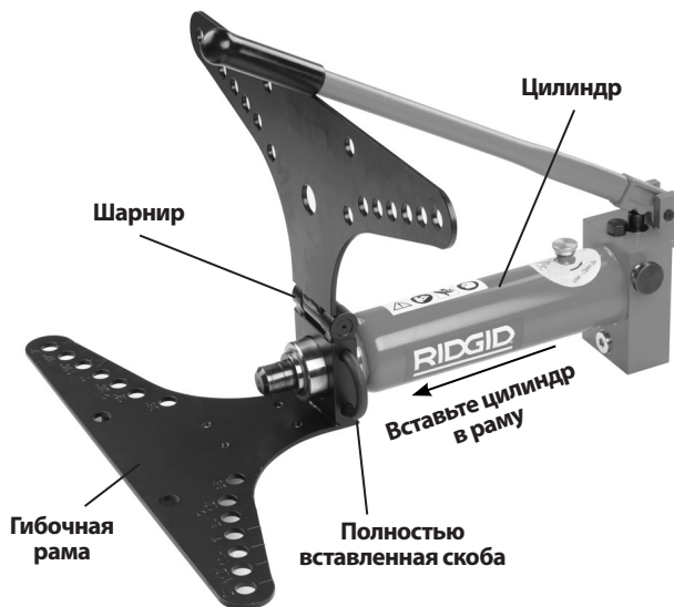
Рис.5 – Сборка 2" и 3" гибочных машин
