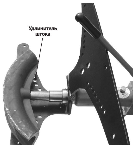
Рис.17 – Установка удлиннителя штока (для лучшей видимости показано в открытом положении без трубы)
